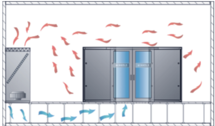
Schéma du principe de refroidissement de salle
